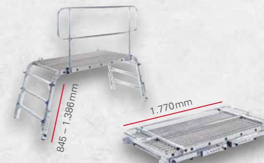
Plataforma de rescate LRP, dimensiones: 1770 x 850 mm, 49 kg, capacidad de carga 500 kg Nº art. 81-73-50
